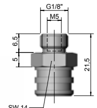
WGS-VNO-G1/8-2 022104
