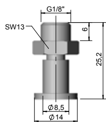
WGS-VNI+G1/8 024045
