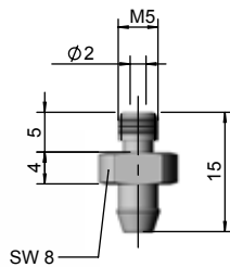
WGS-VN-M5 022048
