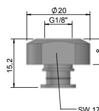
WGS-VNI-G1/8-PI2 024064
