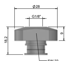
WGS-VNI-G1/8-PI3 024065
