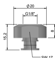
WGS-VNI-G1/8-PI1 024063
