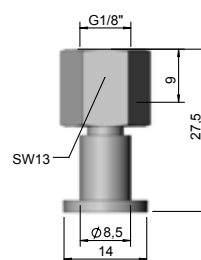
WGS-VNI+G1/8 024045
