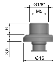
WGS-VNU-G1/8-PI1 024061
