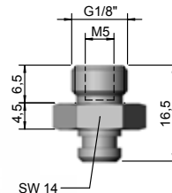
WGS-VNOG1/8-1 022103
