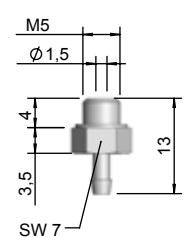
WGS-VNU-M5-PI1 024059
